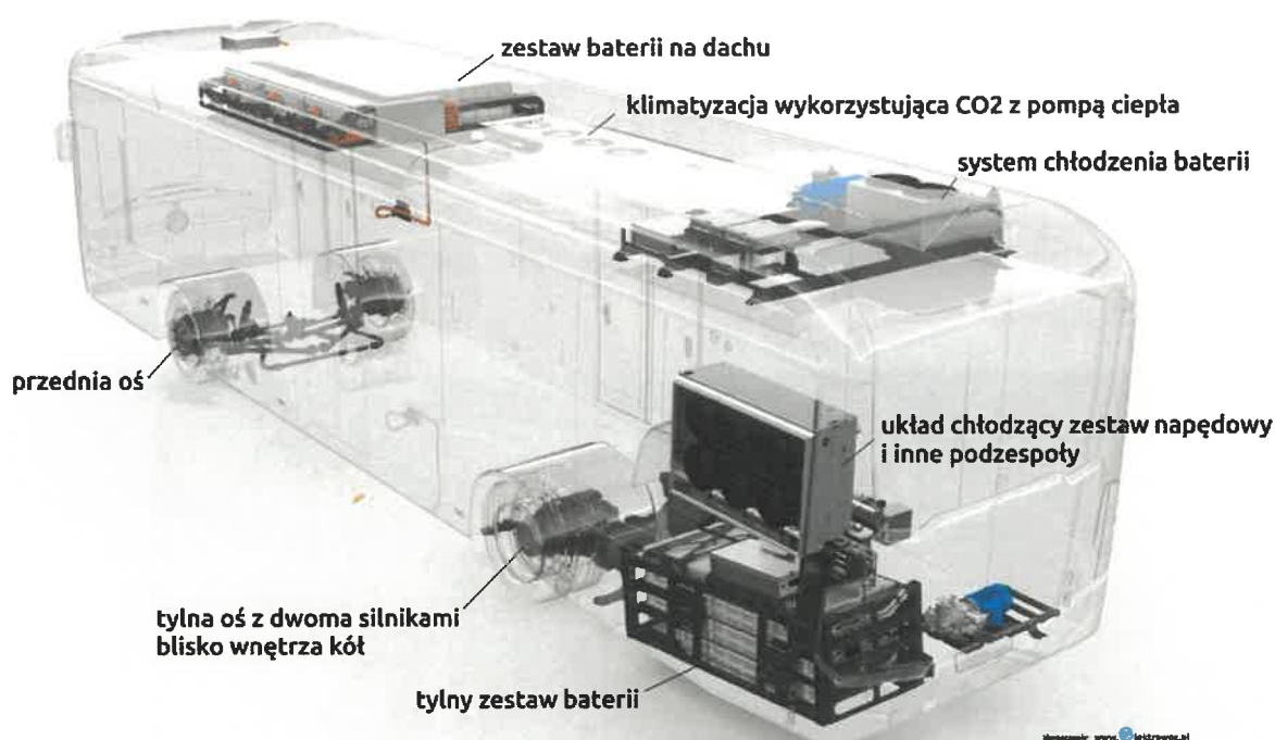
Rysunek 3 Schemat budowy autobusu elektrycznego, źródło: https://elektrowoz.pl/wp-content/uploads/2018/07/Schemat-budowy-elektrycznego-autobusu-eCitaro.jpg
