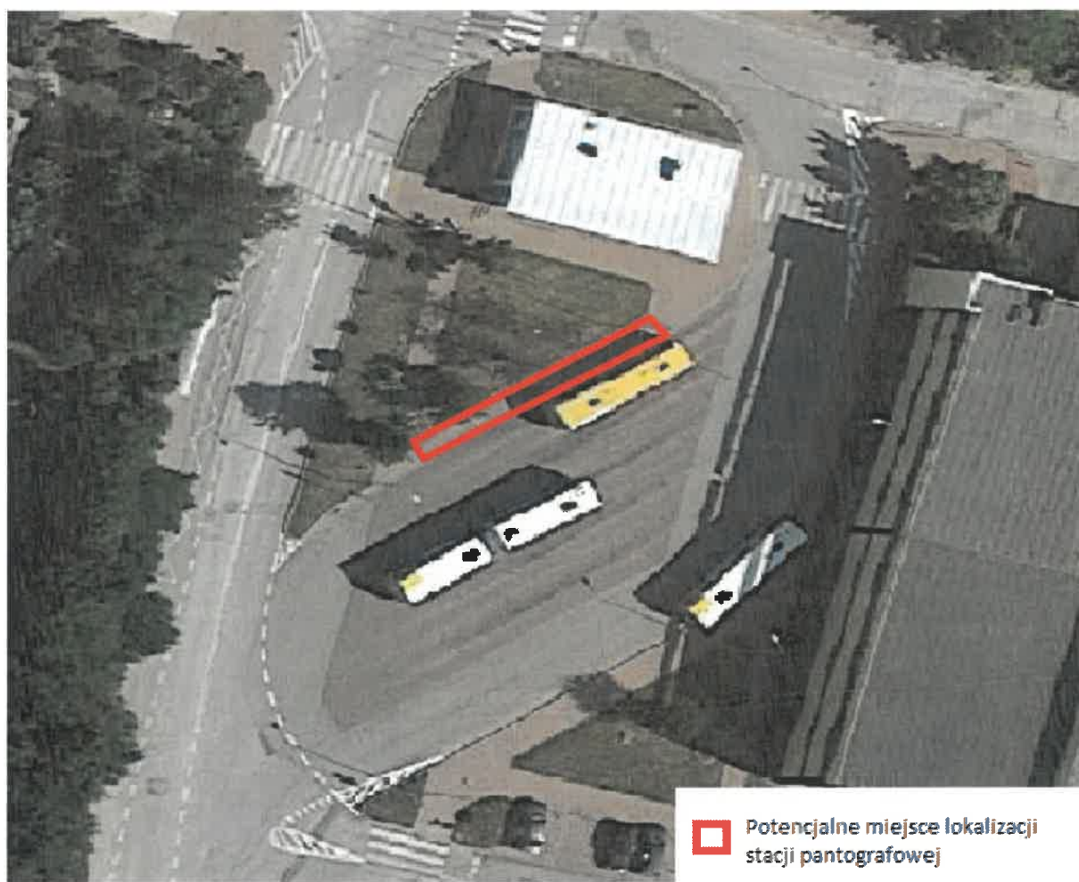
Rysunek 12 Potencjalna lokalizacja stacji pantografowej na mini dworcu komunikacji miejskiej – Osiedle Ślichowice
