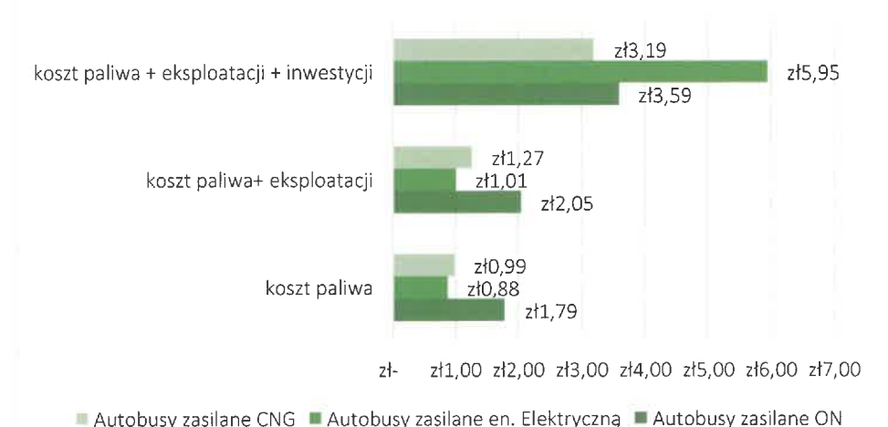
Rysunek 17 Porównanie kosztów jednostkowych w wariantach
